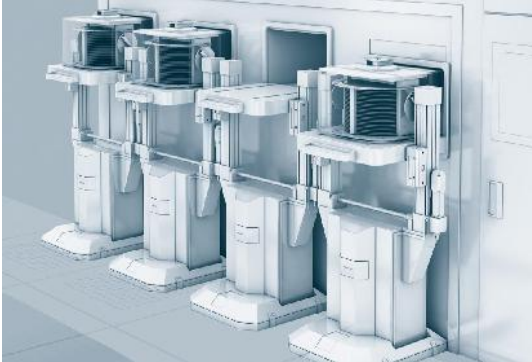
FOUF 清洁 (N2 吹扫)
