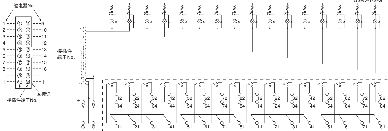
接插件端子配置图 (顶视图)
