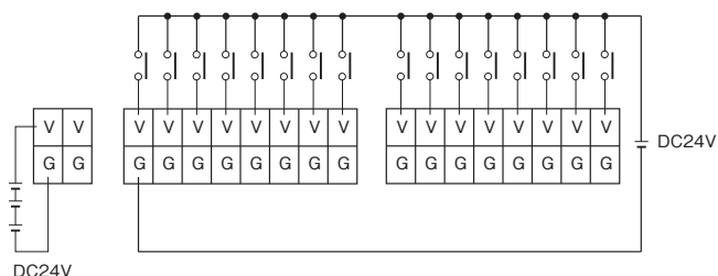
G70V-SID16P-1-C16
